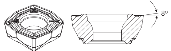
XOKX-MS Sisäpala
