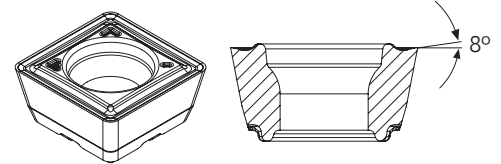
XOKX-MS Sisäpala
