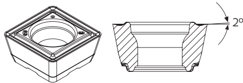
XOKX-MP Sisäpala
